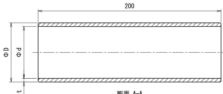
断面 A-A
